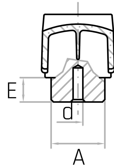
Mod. MH-PGR
